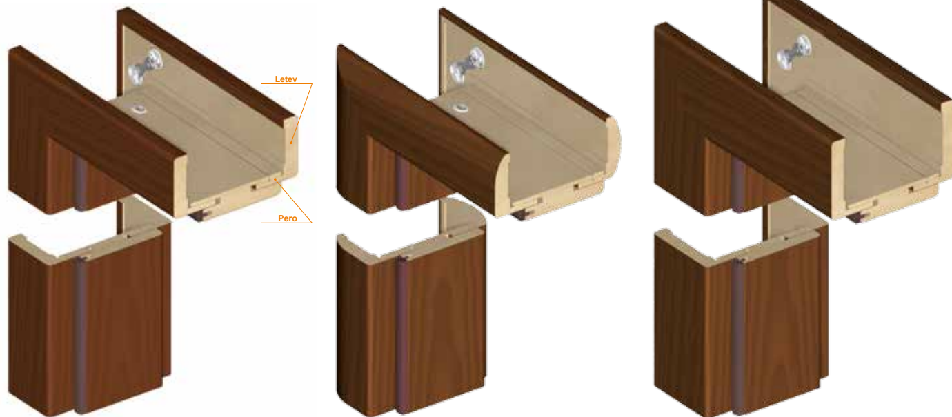
ORS1 Nastavljiv podboj z ravno letvijo širine 60 mm
